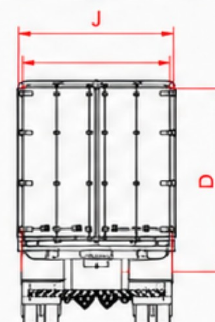
VISTA TRASEIRA
